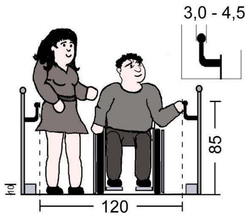
Rampe, Querschnitt
